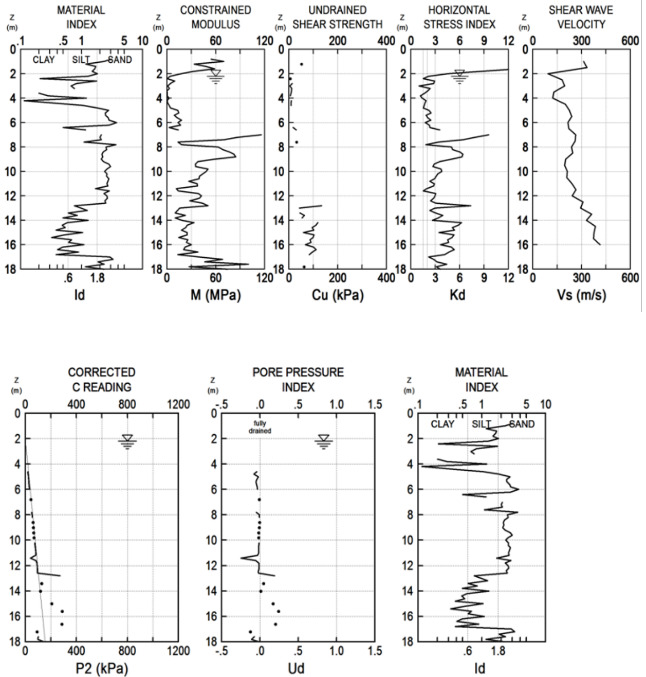
Fig. 32. DMT results, A3.
