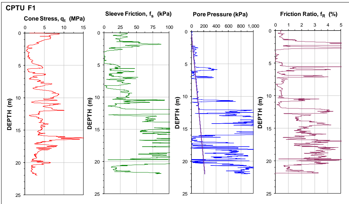
Fig. 27. Results of CPTU F1.
