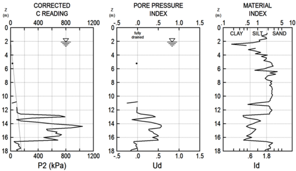
Fig. 36. DMT results, F1.
