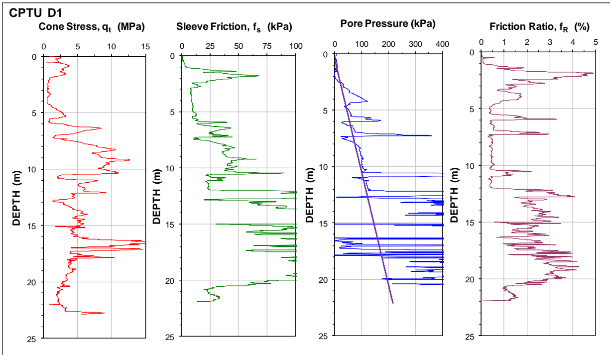
Fig. 23. Results of CPTU D1.
