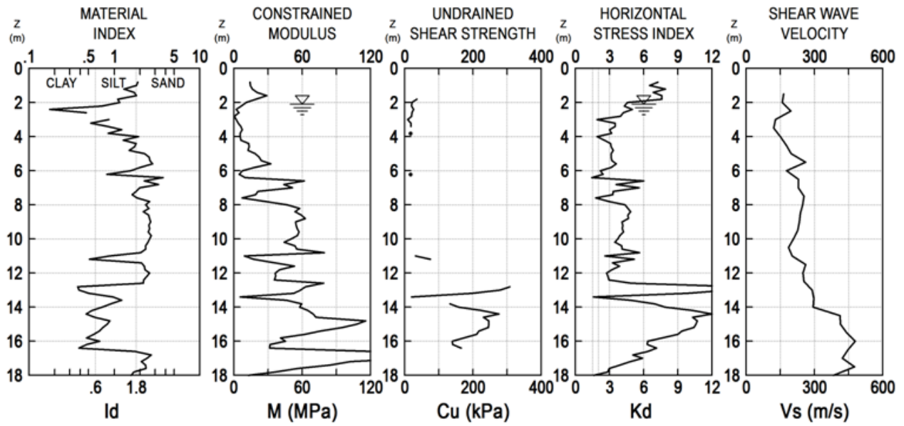
Fig. 35. DMT results, F1.
