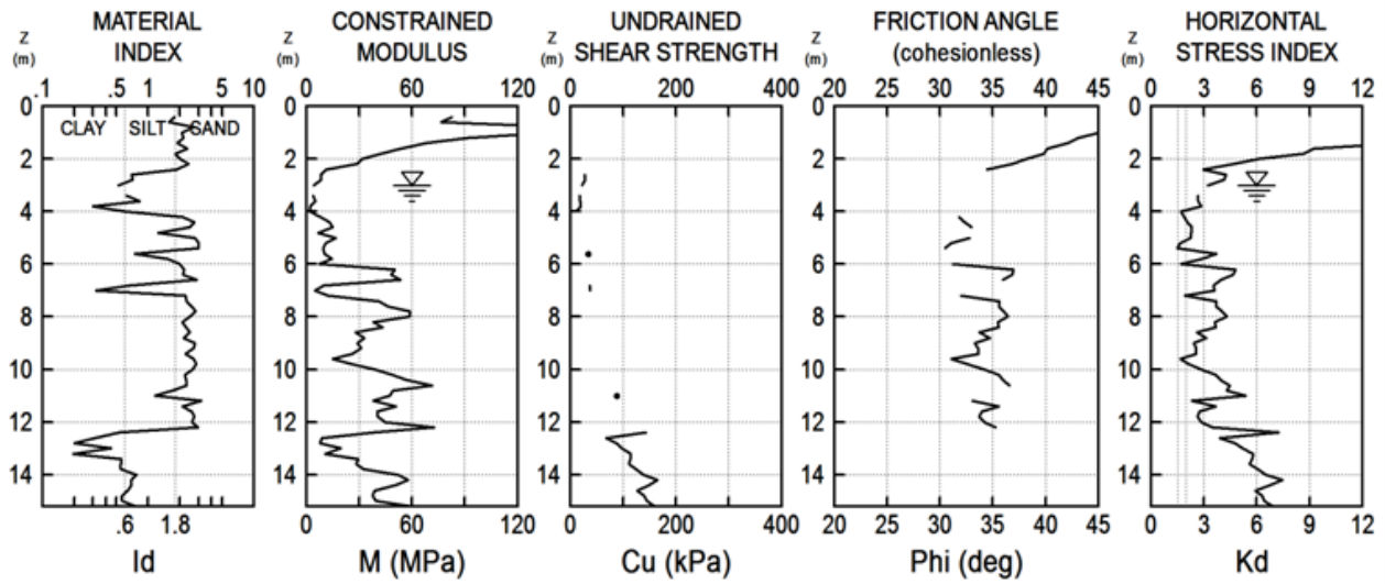
Fig. 37. DMT results, D1.
