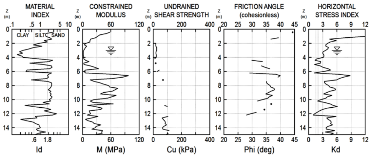
Fig. 38. DMT results, E2.
