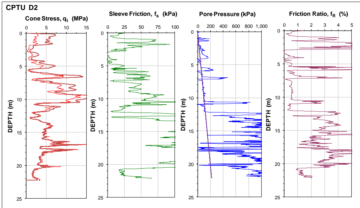
Fig. 24. Results of CPTU D2.
